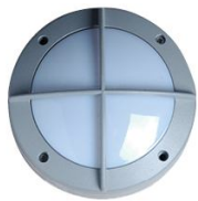
HC-FCD-7208 功率：12W 电压：85-265V 尺寸：Φ220×80mm
