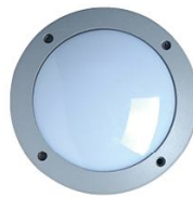
HC-FCD-7210 功率：12W 电压：85-265V 尺寸：Φ220×80mm
