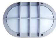
HC-FCD-7206 功率：10W 电压：85-265V 尺寸：220×135×55mm
